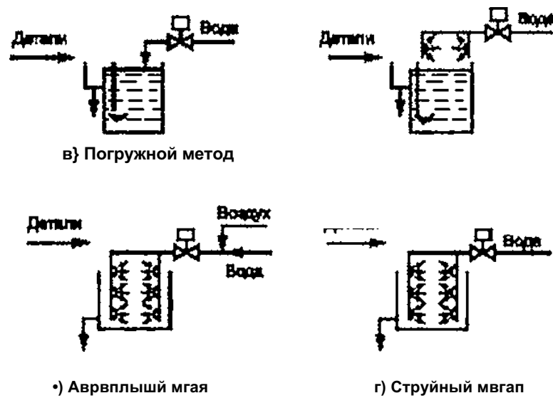
Рисунок 1 — Методы промывок
