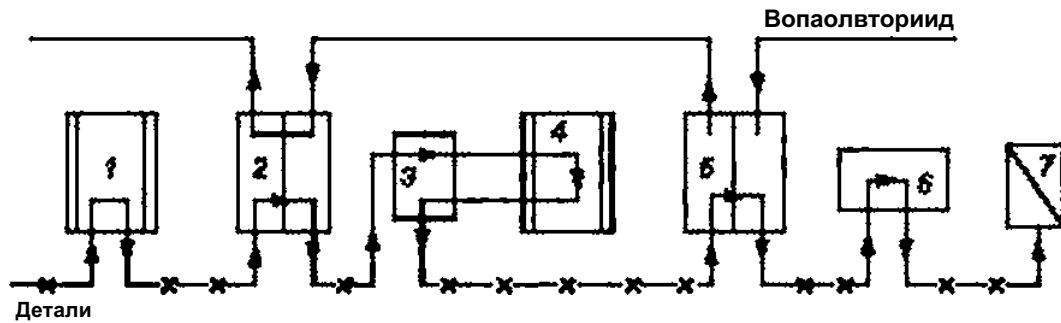
Рисунок Б.2 — Схема промывки деталей, покрываемых металлами, не способными к контактному выделению (подача воды и перемещение деталей)
